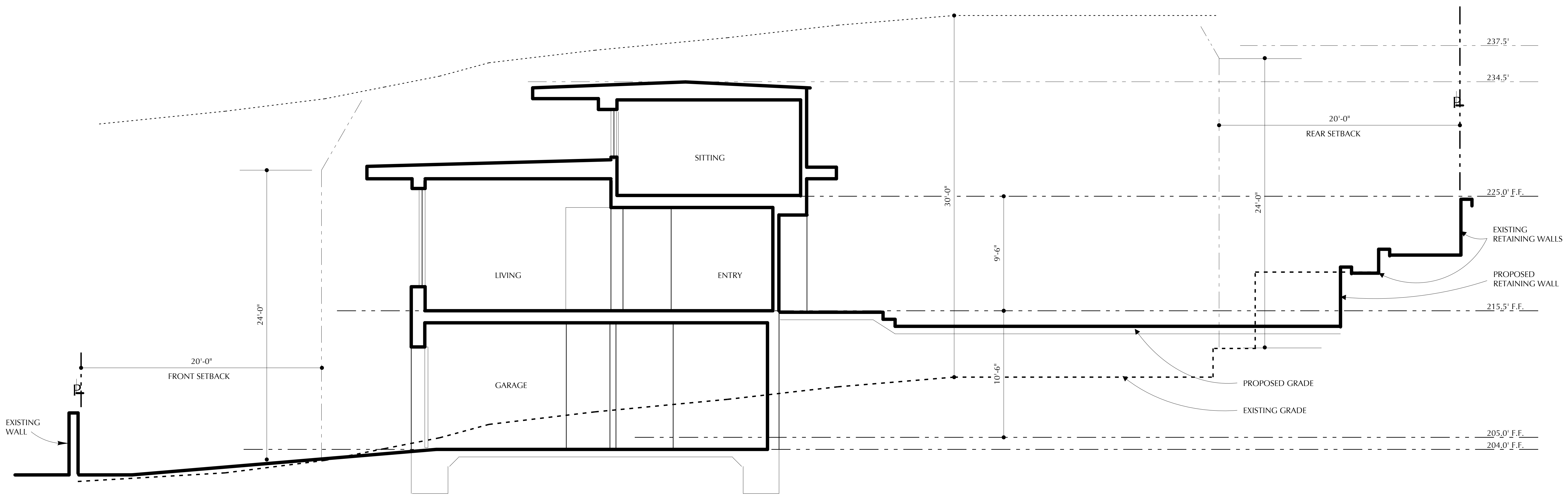
SECTION 'B-B'
